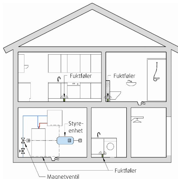
Systemskisse for VIWA Watersafe trådløs lekkasjestopper.
